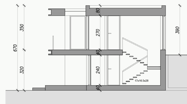
SNITT B-B
