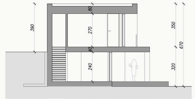
SNITT B-B
