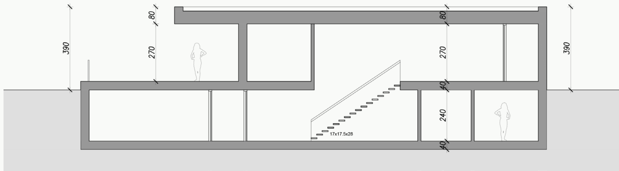
SNITT A-A
